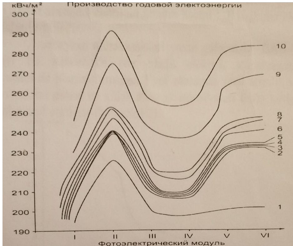
Şəkil 1. Fotoelektrik modullar üzrə illik elektrik enerjisinin istehsalının proqnozu
