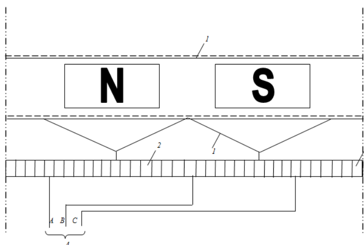
Рис. 1. Схема соединения якорной обмотки. N, S – магнитные полюсы; 1 – обмотка; 2 – коллекторные пластины; 3 – коллектор; 4 – зажимы обмотки возбуждения.
