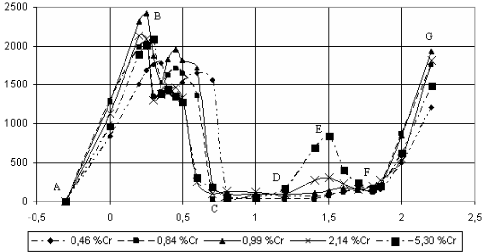
Şəkil 1. Müxtəlif ərintilərin qütbləşmiş anod əyriləri – 1 M H_2SO_4
