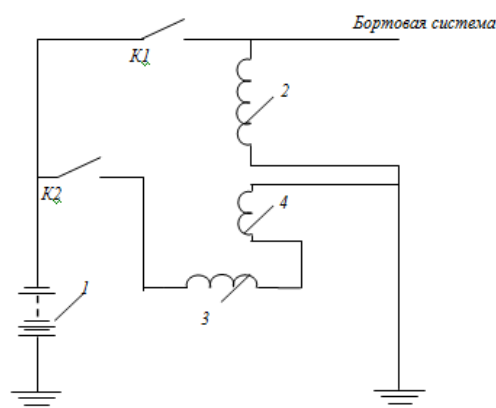
Рис. 2. Электрическая схема стартер-генератора в режиме стартера. 1 – аккумуляторная батарея; 2 – шунтовая обмотка возбуждения; 3 – якорная обмотка; 4 – последовательная обмотка возбуждения; K1 – контакт для включения бортовую сеть на аккумуляторную батарею; K2 – контакт пускового реле
