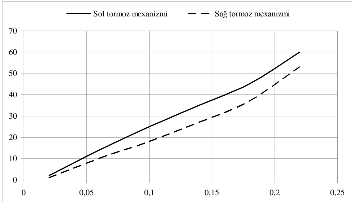
Şəkil 2. Tormoz mexanizminin qeyri-bərabərlik əmsalının friksion cütlərin sürtünmə əmsalından asılılığı
