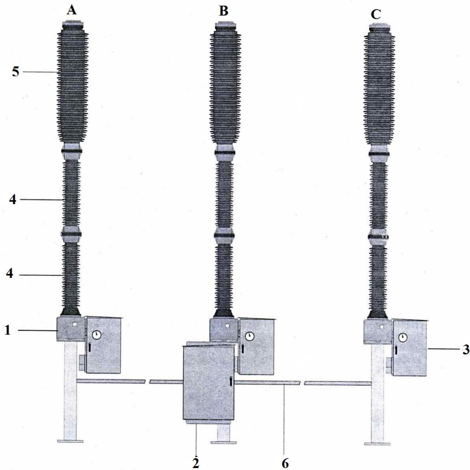
Şəkil 1. 3AP 1 F1 güc açarının quraşdırılması.
