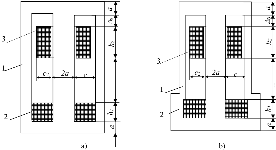
Şəkil 1. Qida gərginliyinin U_1=U_{\max} qiyməti üçün levitasiya dolağının vəziyyəti a-düz maqnit sistemi; b- pilləvari maqnit sistemi
