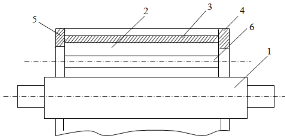
Рис. 1. Конструктивная схема рабочего ротора
