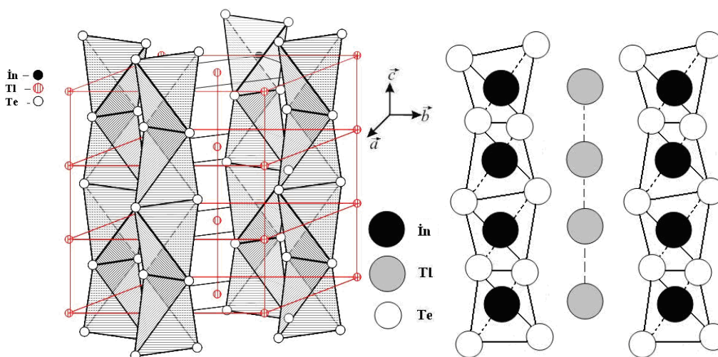
Şəkil 1. TlInTe 2 kristalının quruluşu
