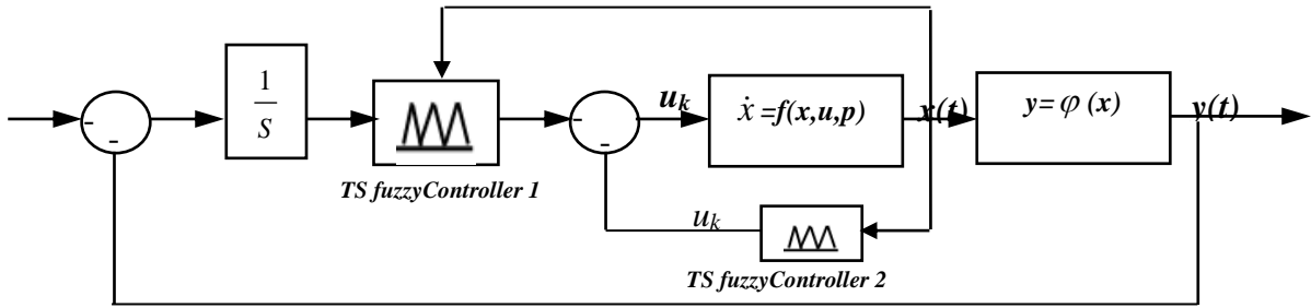
Şəkil 1. Əks əlaqəli TS tipli qeyri-səlis modellə təsvir olunan qeyri-xətti dinamik obyektlərin idarəetmə sisteminin ümimiləşdirilmiş struktur sxemi
