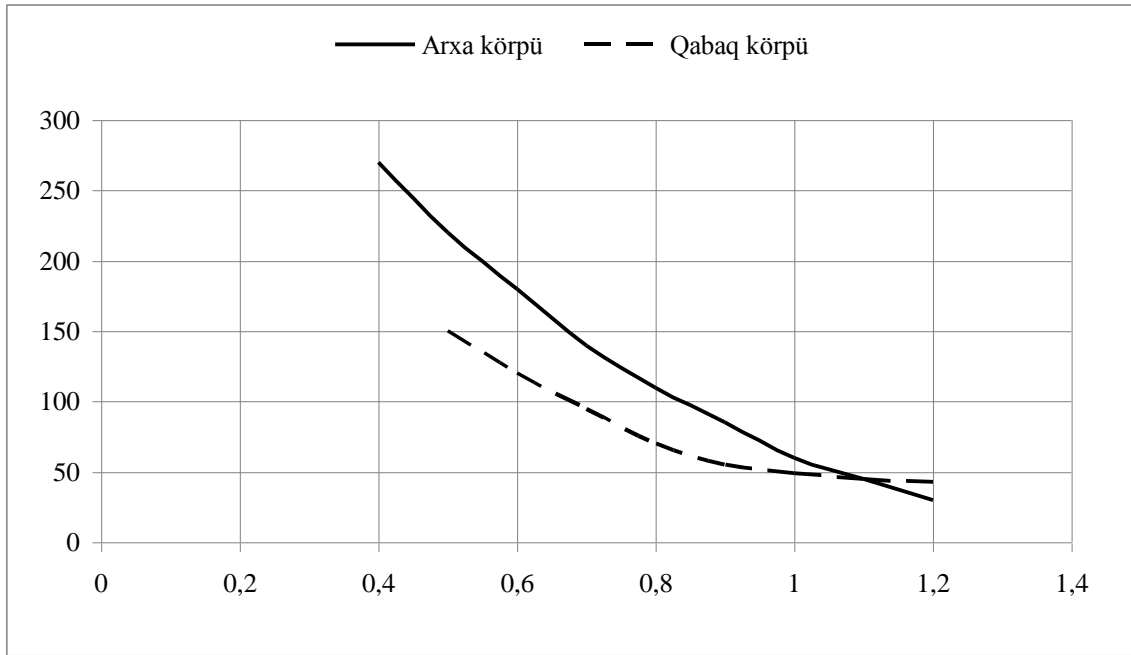
Şəkil 1. KAMAZ -5511 avtomobilinin tormoz momentinin tormoz barabanı ilə üstlük arasında araboşluğundan asılılığı
